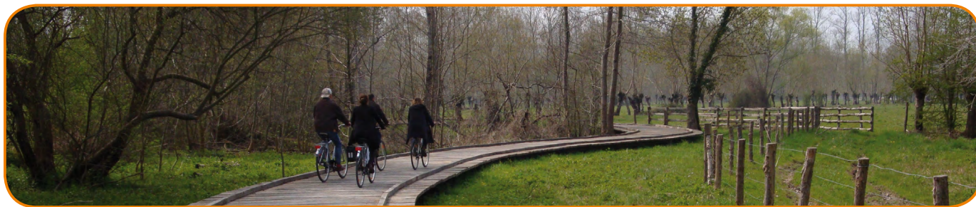
Platelage bois avec chasse-roues (Marais poitevin)
